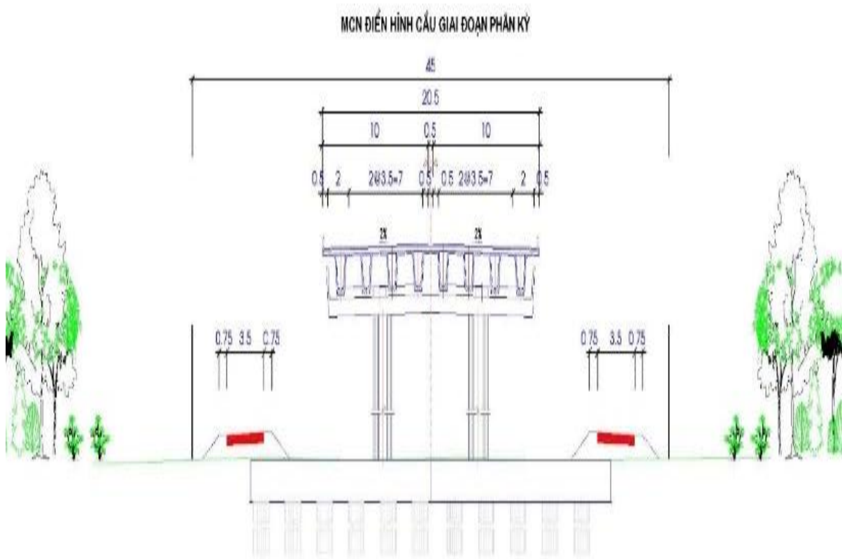
Mặt cắt điển hình Cầu Mã Đà giai đoạn phân kỳ đầu tư
