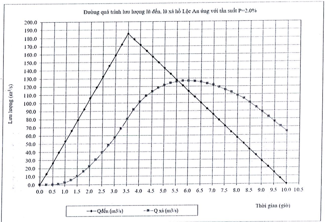
Hình 4. 2: Quá trình lũ đến, lũ xả ứng với tần suất P=2,0%
