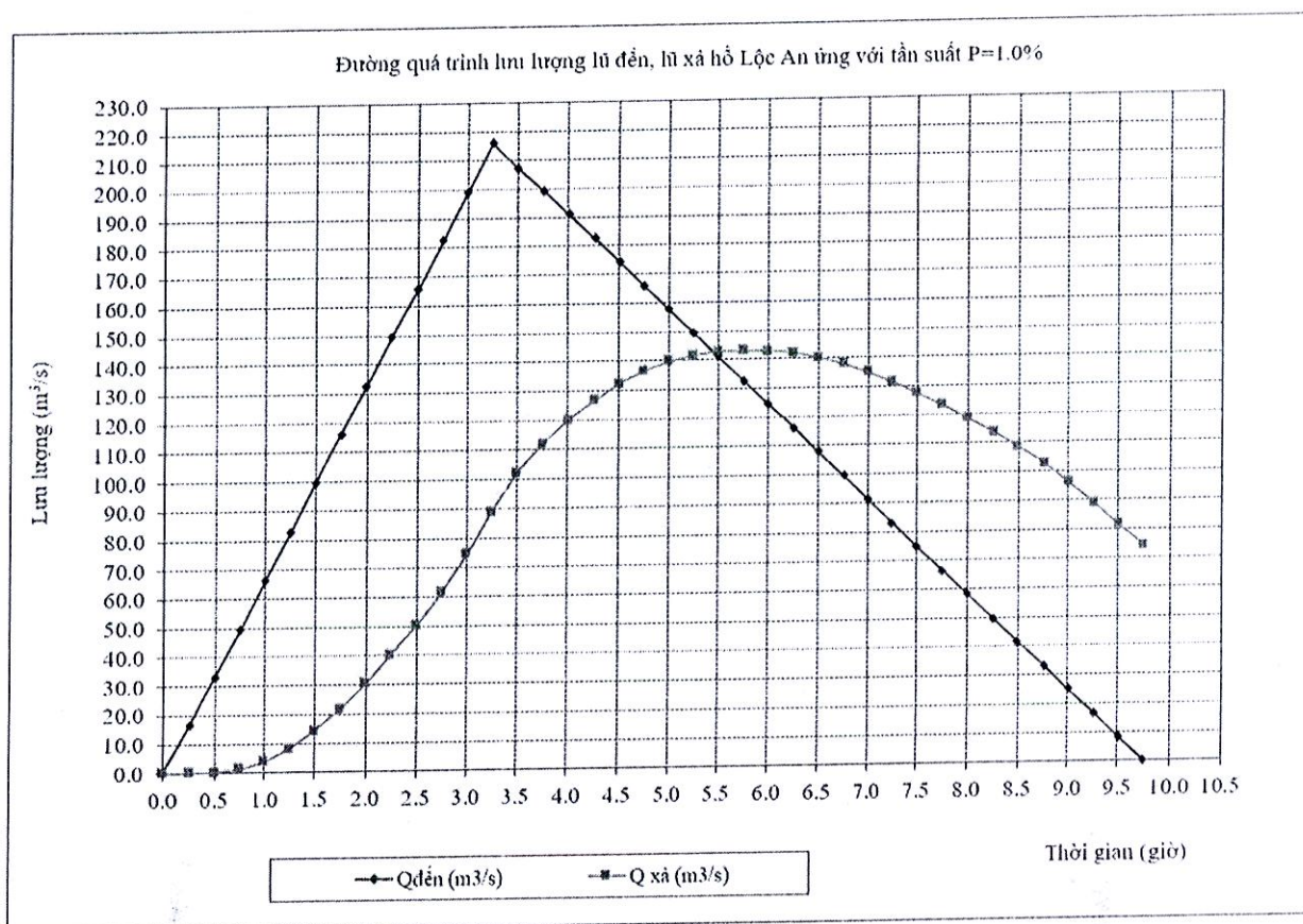
Hình 4. 3: Quá trình lũ đến, lũ xả ứng với tần suất P=1,0\%
