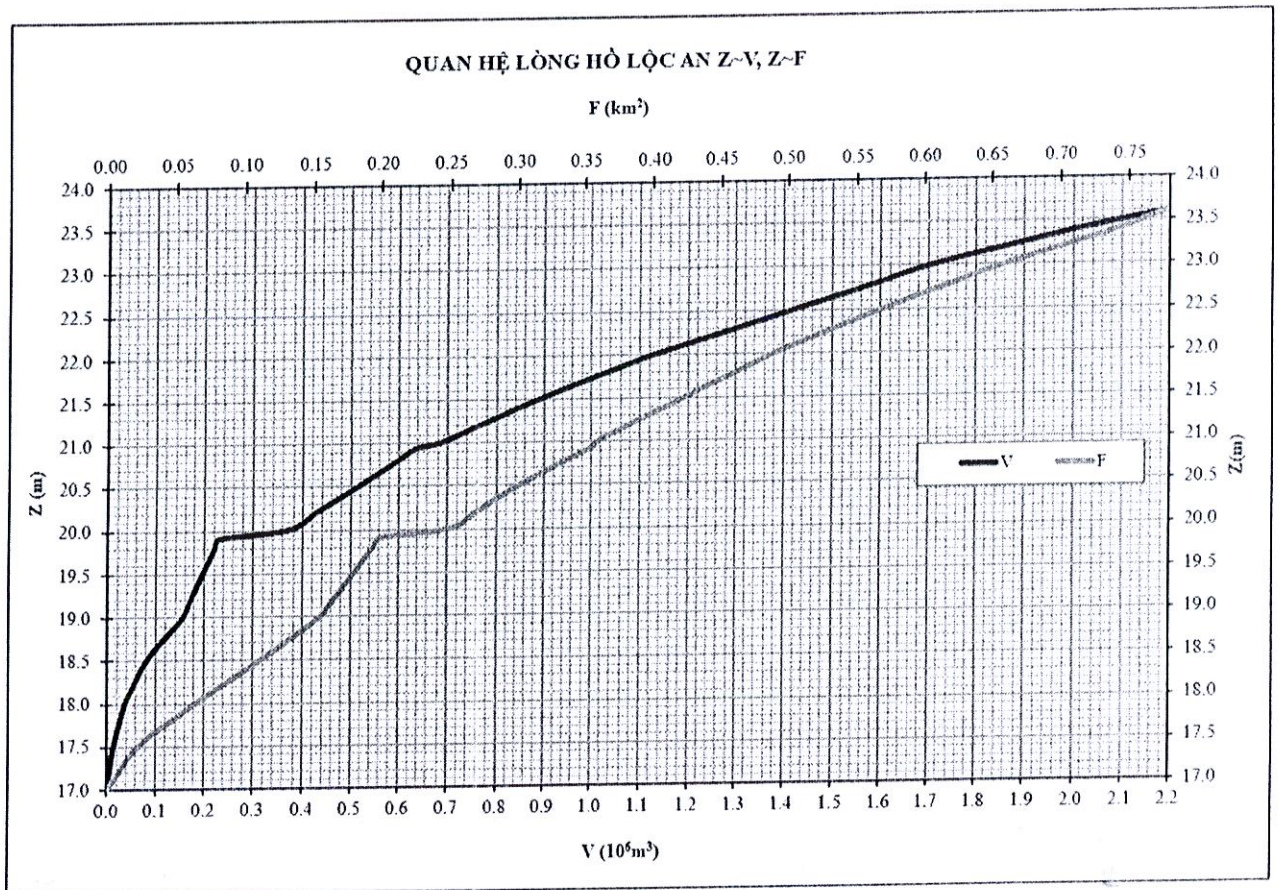
Hình 4. 1: Đường quan hệ lòng hồ chứa nước Lộc An
