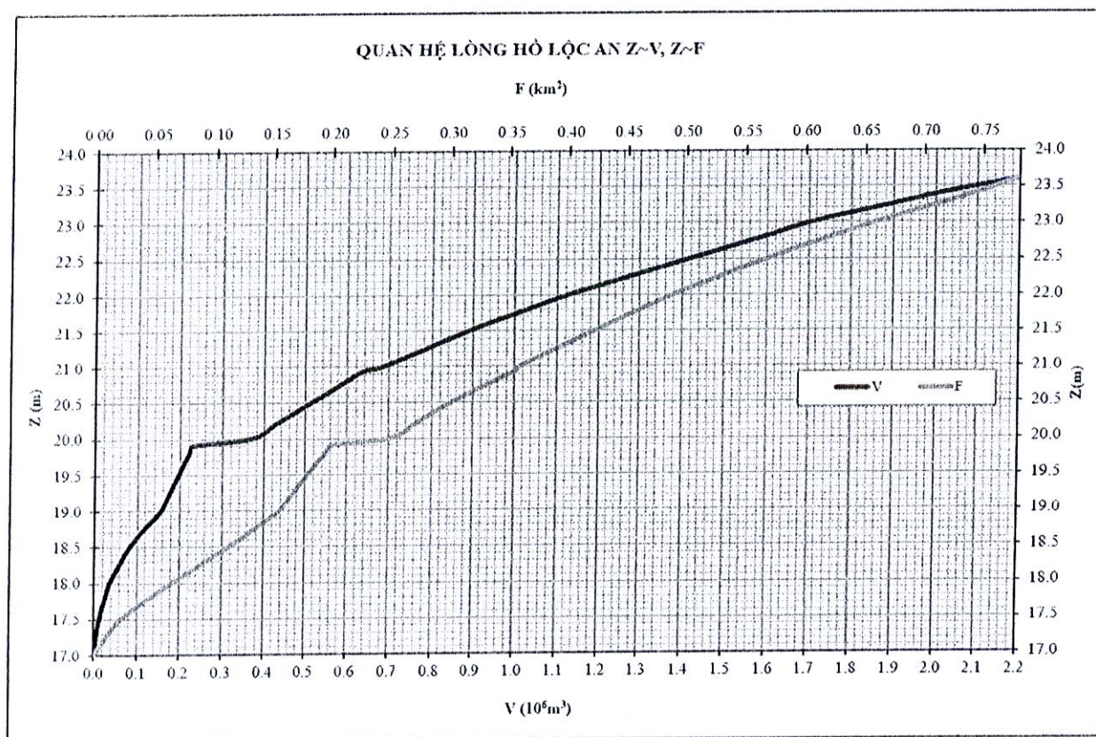
Hình 4: Quan hệ Z-V, Z-F
