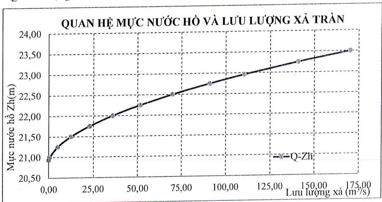
Hình 6. 1: Quan hệ giữa lưu lượng qua tràn Q và mực nước hồ Z
