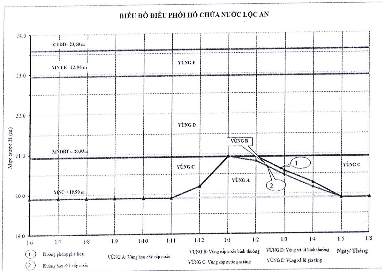
Hình 5. 1: Biểu đồ điều phối hồ chứa nước Lộc An
