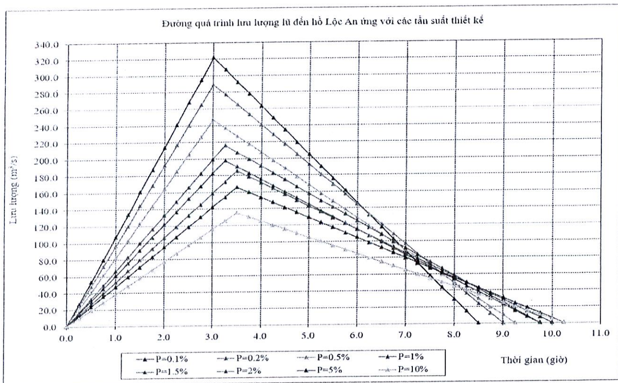
Hình 3. 1: Quá trình lũ đến lưu vực hồ chứa nước Lộc An ứng với các tần suất thiết kế
