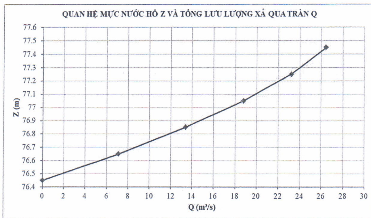
Hình 2: Quan hệ Z - Q tràn xả lũ hồ Suối Đầm
