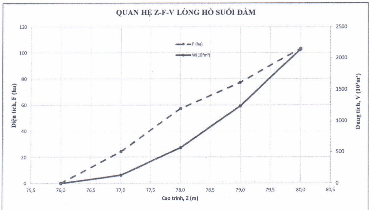
Hình 4: Biểu đồ quan hệ Z \sim V \sim F hồ Suối Đầm
