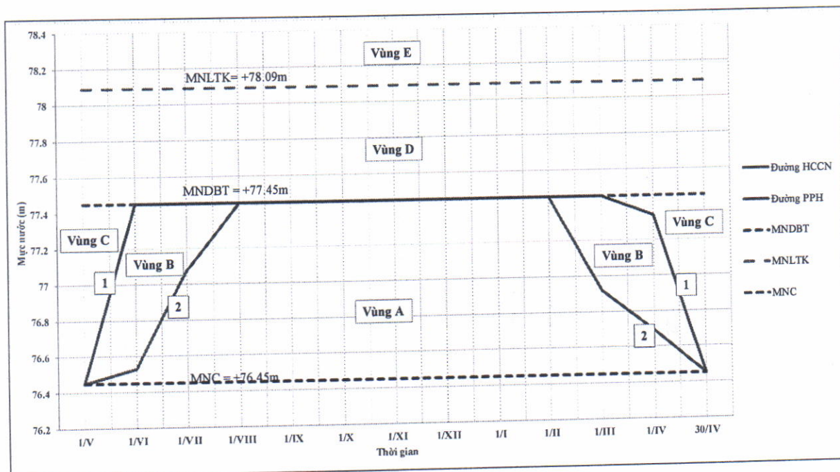
Hình 1: Biểu đồ điều phối hồ chứa
